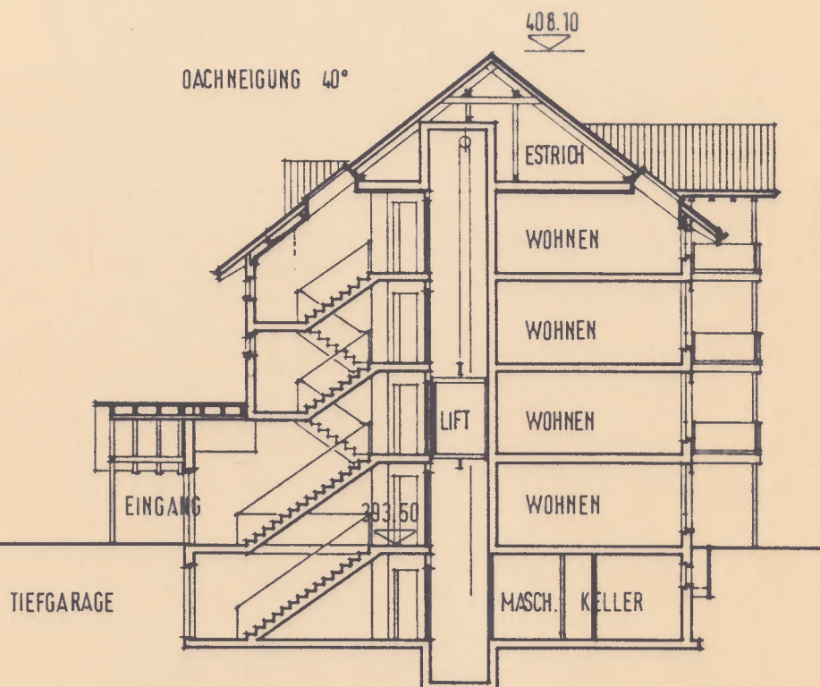
GEBÄUDEQUERSCHNITT
