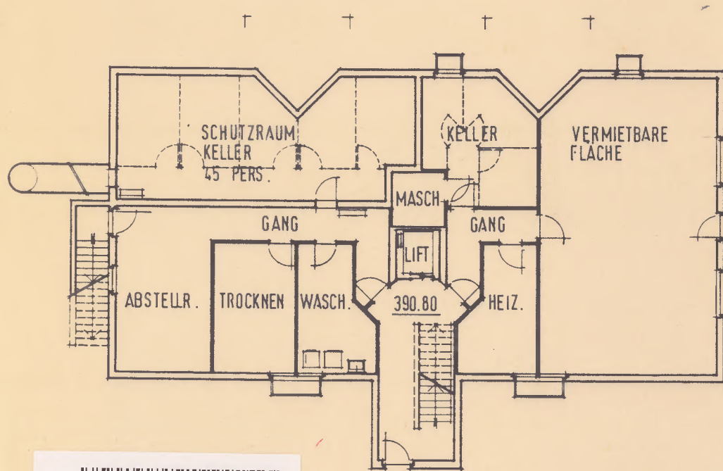
GRUNDRISS UNTERGESCHOSS
