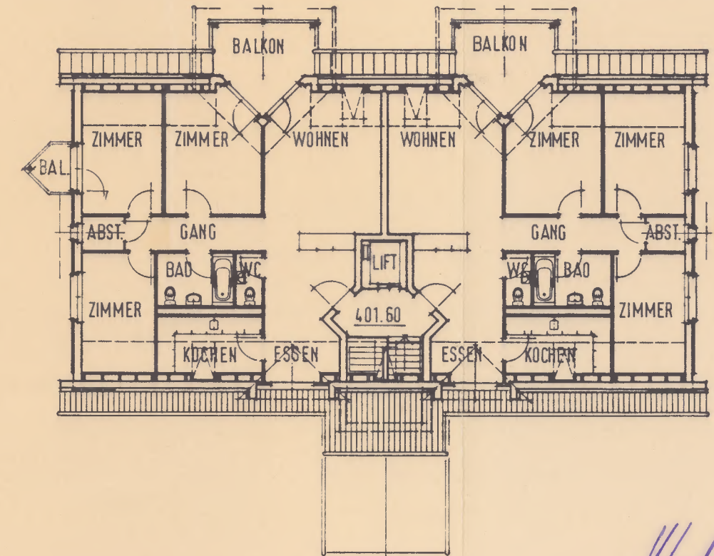
GRUNDRISS DACHGESCHOSS
