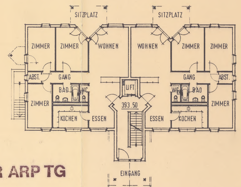
GRUNDRISS ERDGESCHOSS
