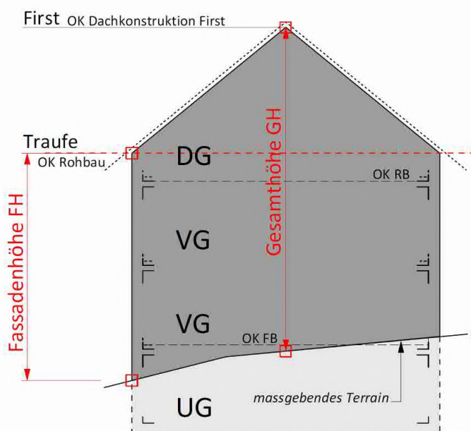
Schrägdach
