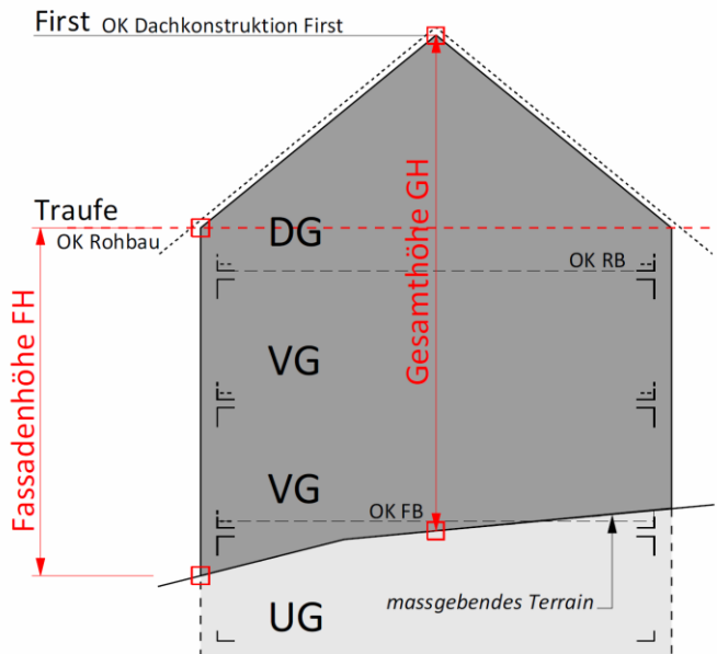
Schrägdach
