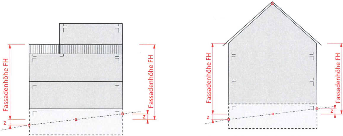
Hangzuschlag z maximal 1.50 m bei geneigtem Terrain > 12 %
