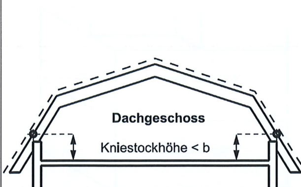
b zulässiges Mass für die Kniestockhöhen von Dachgeschossen
