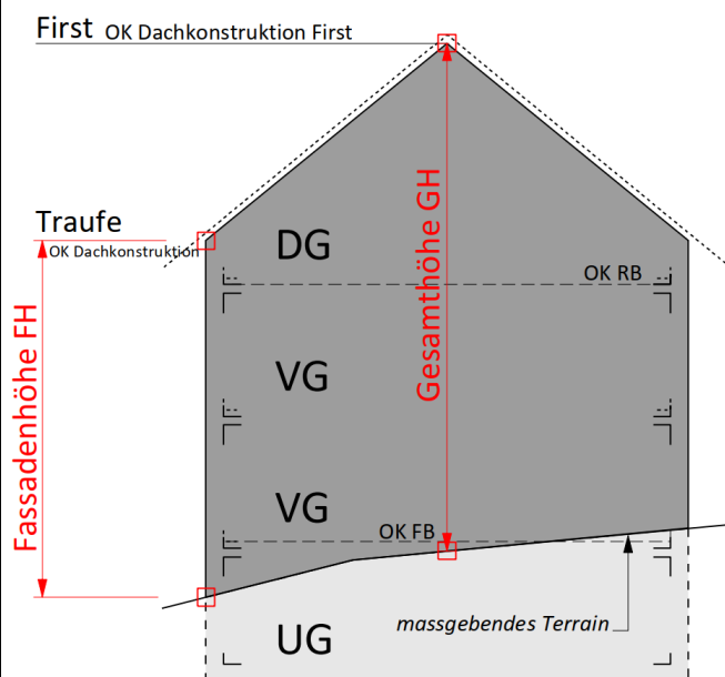
Schrägdach
