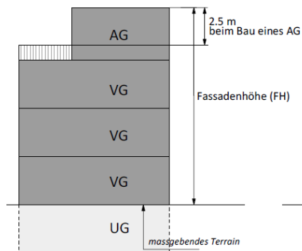
Massskizze Fassadenhöhen
