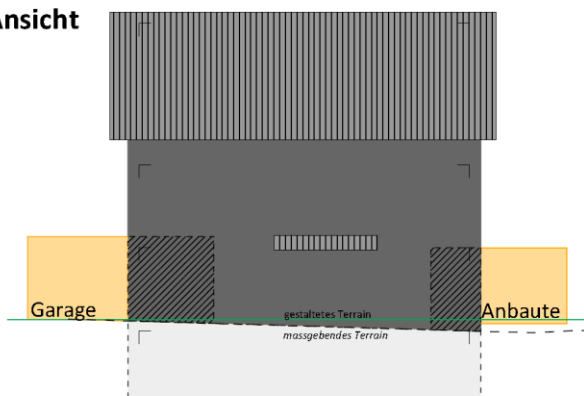
Ansicht
