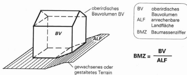
Beispiel Schrägdach:
