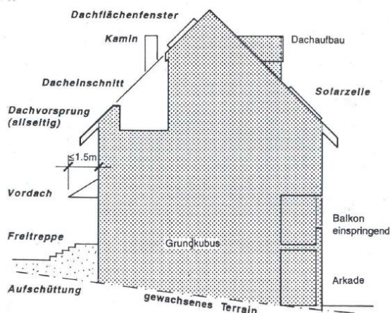
Beispiel Schrägdach:
